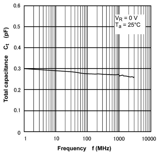
Fig. 9.4 C_t - f
