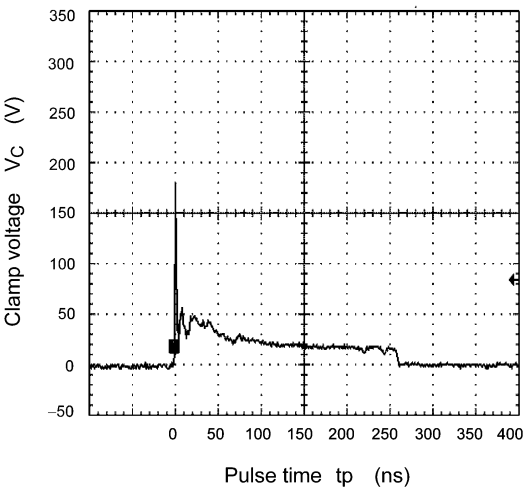
Fig. 6.1.1 +8 kV
