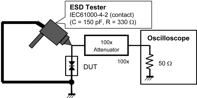
Fig. 6.1.3 IEC61000-4-2 (Contact)
