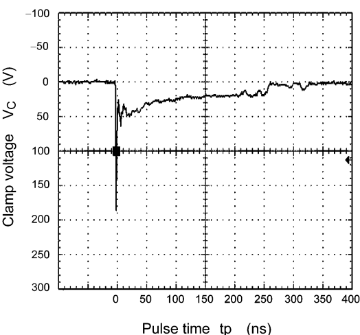
Fig. 6.1.2 -8 kV
