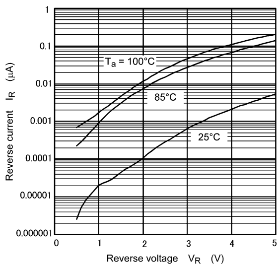
Fig. 9.2 I_R - V_R
